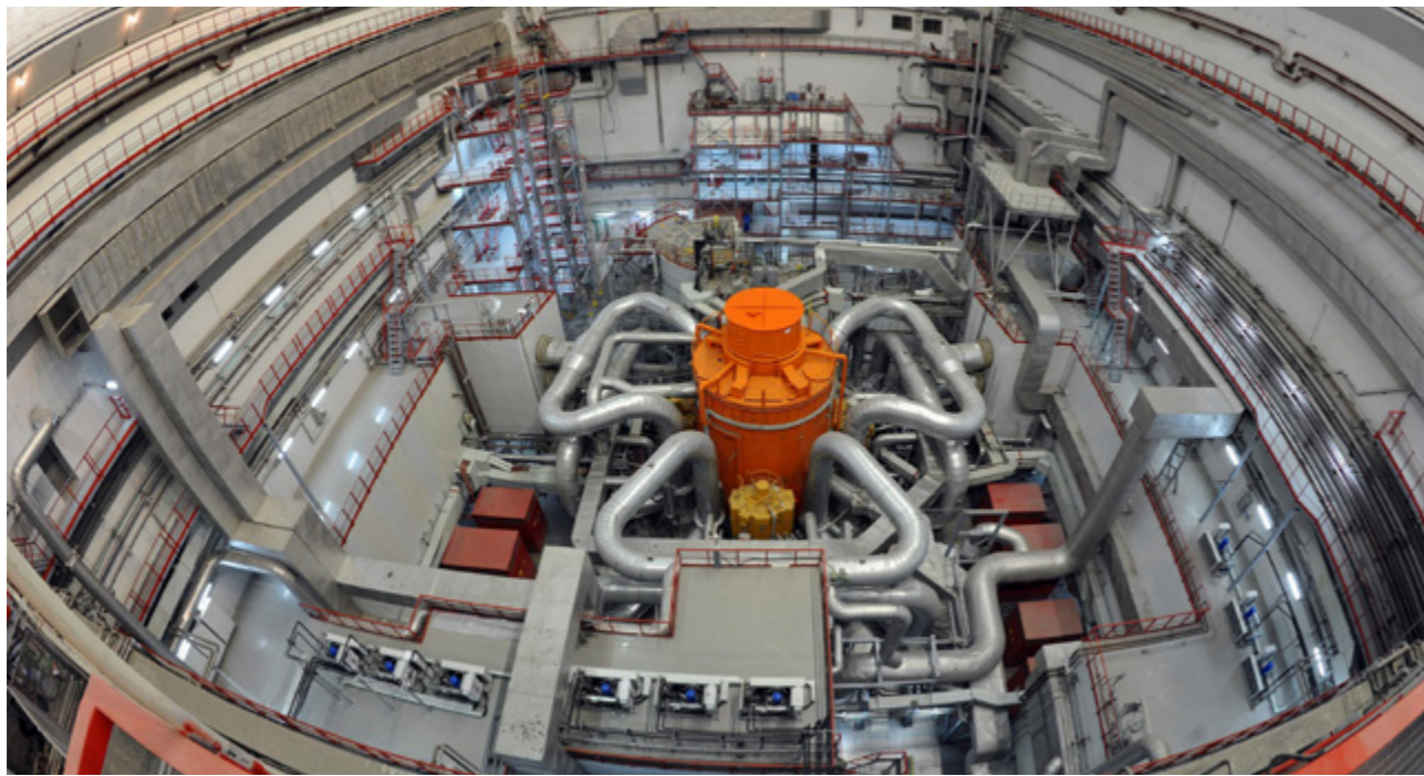
Центральный зал реакторного отделения БН-800. Фото предоставлено Концерном «Росэнергоатом», http://stock.rosenergoatom.ru/
